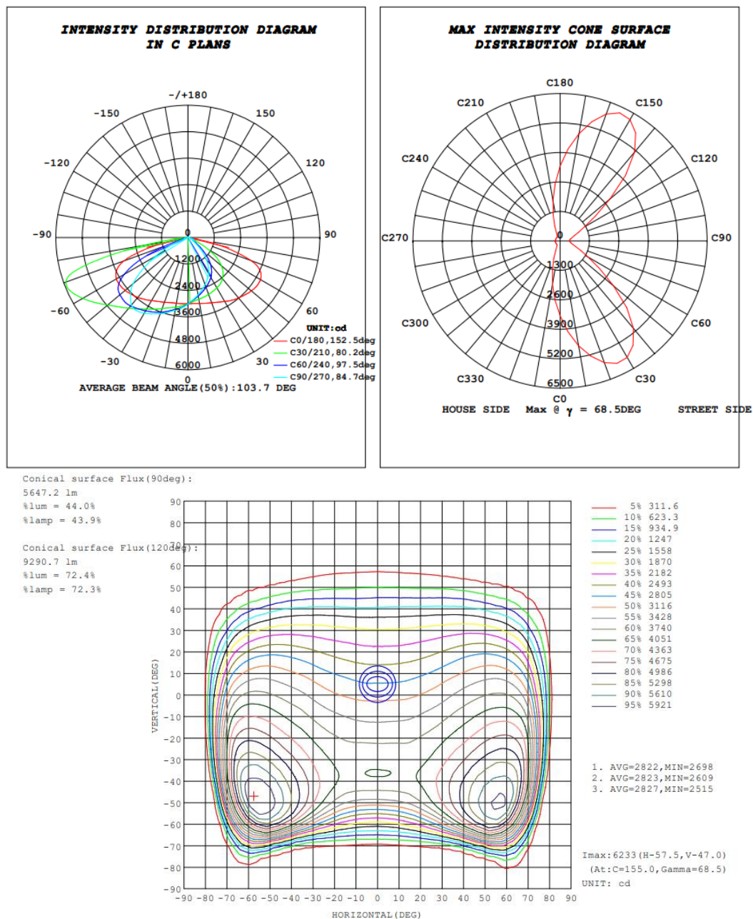
Figura 03 – Curvas - Amostra 01
