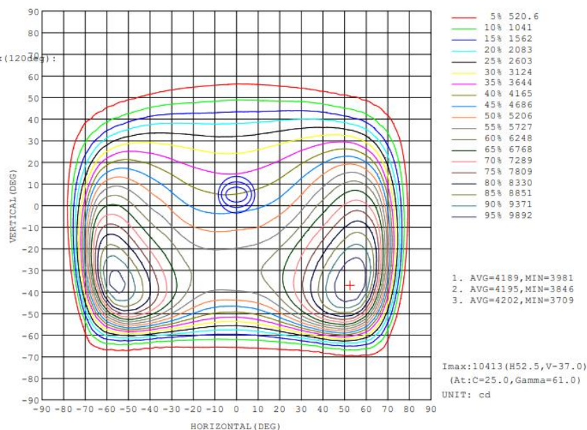
Figura 05 – Curvas - Amostra 03
