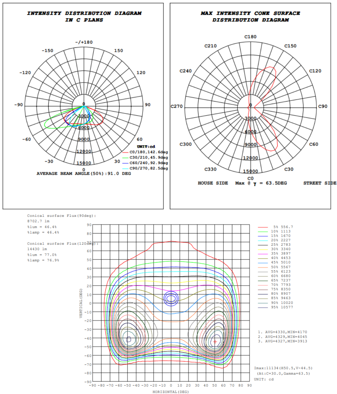
Figura 03 – Curvas - Amostra 01
