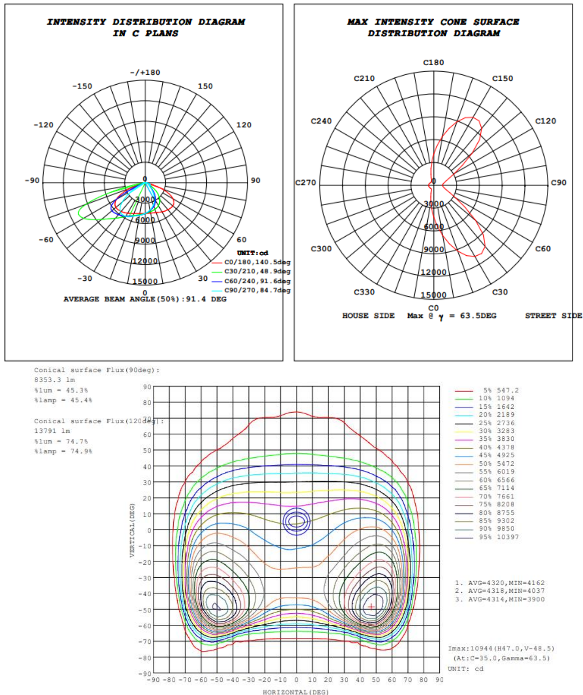
Figura 04 – Curvas - Amostra 02
